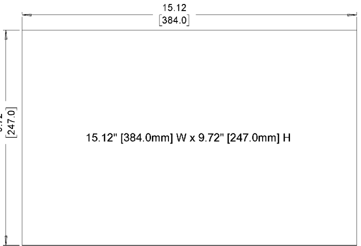
Cutout Dimensions
